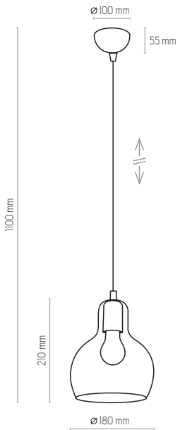
588 | MANGO | 1 x E27, max 60W | KL 7806
