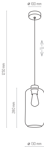
2077 | MARCO | 1 x E27, max 60W | KL 7409
