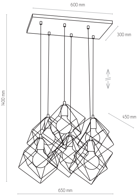
2779 | ALAMBRE | 6 x E27, max 60W | DM 50A / DM 50B
