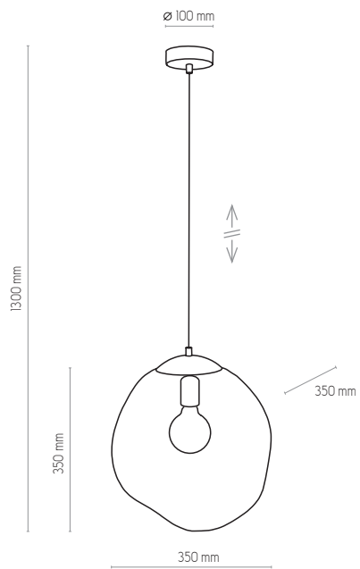
4262 | SOL | 1 x E27, max 60W | KL 7433
