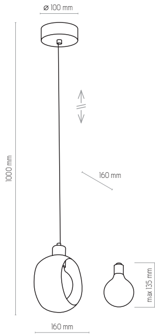
2741 | CYKLOP WHITE | 1 x E27, max 60W
