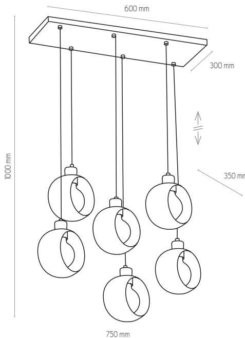
2746 | CYKLOP WHITE | 6 x E27, max 60W
