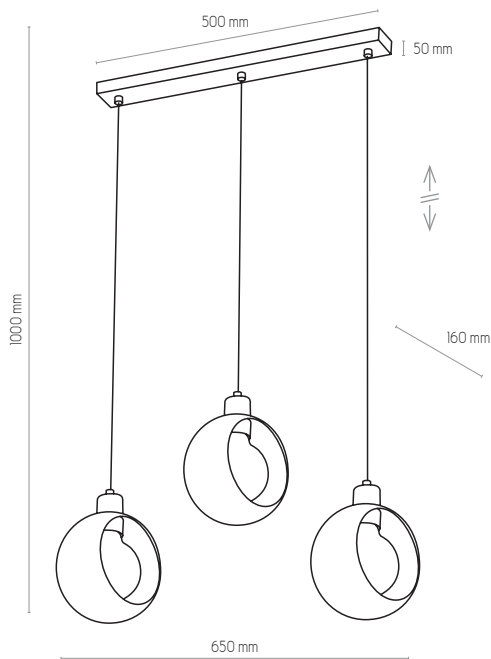
2743 | CYKLOP WHITE | 3 x E27, max 60W
