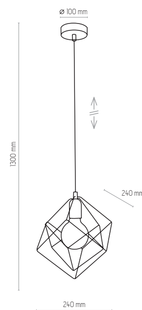
2777 | ALAMBRE | 1 x E27, max 60W | DM 50A / DM 50B
