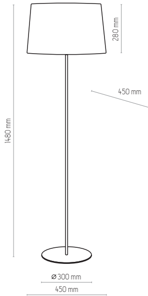
2920 | MAJA BLACK | 1x E27, 25W LED | AB 8404
