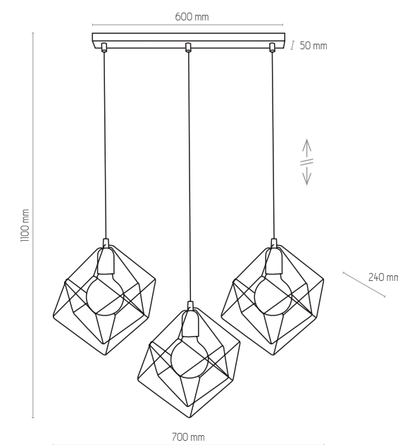
2699 | ALAMBRE | 3 x E27, max 60W | DM 50A / DM 50B
