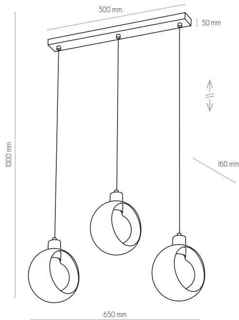
2753 | CYKLOP BLACK | 3 x E27, max 60W
