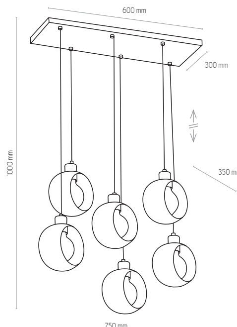
2756 | CYKLOP BLACK | 6 x E27, max 60W
