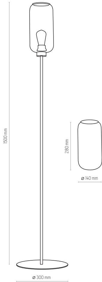
5052 | MARCO | 1 x E27, max 60W | KL 7409
