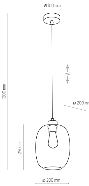
3180, 3181, 3182, 3183 | ELIO | 1 x E27, max 60W
