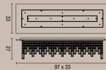
plafoniera rettangolare Frangia grande Frangia large rectangular ceiling lamp 2184
