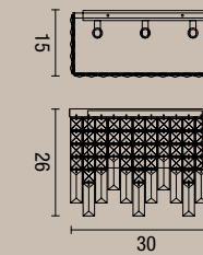
applique Frangia rettangolare Frangia rectangular wall lamp 2231
