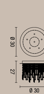
plafoniera tonda Frangia piccola Frangia small round ceiling lamp 2188
