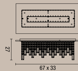
plafoniera rettangolare Frangia grande Frangia large rectangular ceiling lamp 2183
