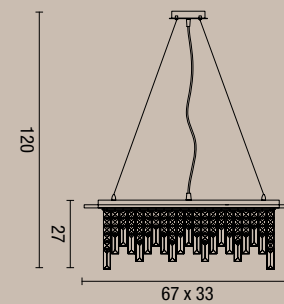
sospensione Frangia piccola Frangia small pendant lamp 2194
