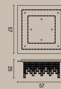
plafoniera quadrata Frangia grande Frangia large square ceiling lamp 2196
